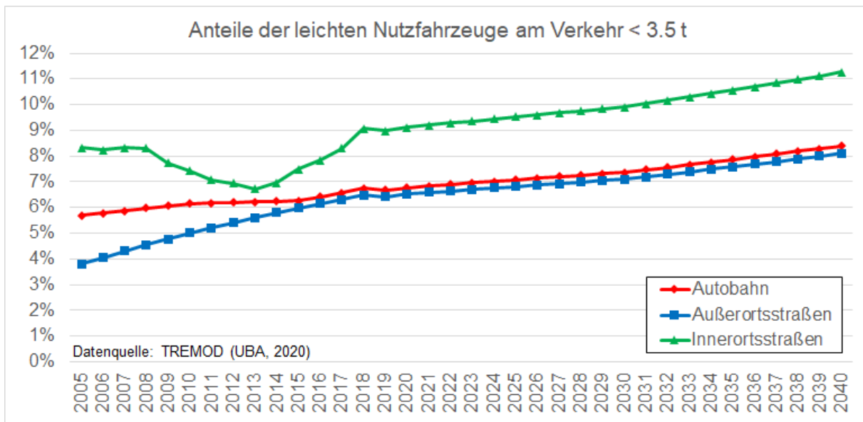
Abbildung 1: In RLuS berücksichtigter Anteil leichter Nutzfahrzeuge kleiner 3,5 t zulässiger Gesamtgewichts am Verkehr.
