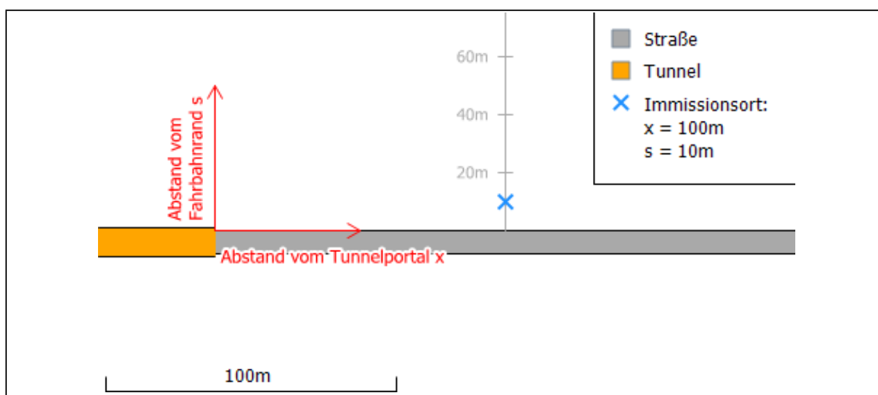
Abbildung 4: Lageplan eines Tunnelportals.
