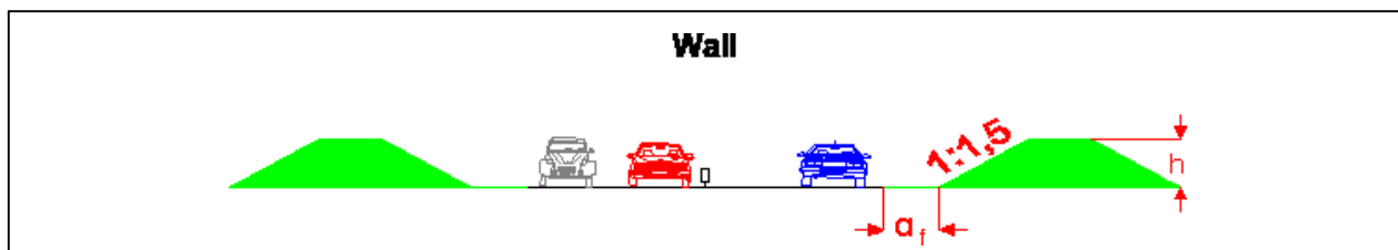
Abbildung 7: Querschnitt für den Lärmschutzwand. Lärmschutzwälle auf beiden Straßenseiten, die immissionsseitig gleich behandelt werden.
