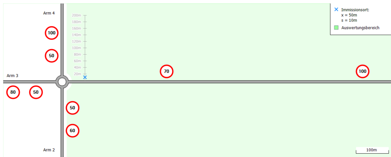
Abbildung 9: Lageplan für einen Kreisverkehr. Näheres s. Text.
