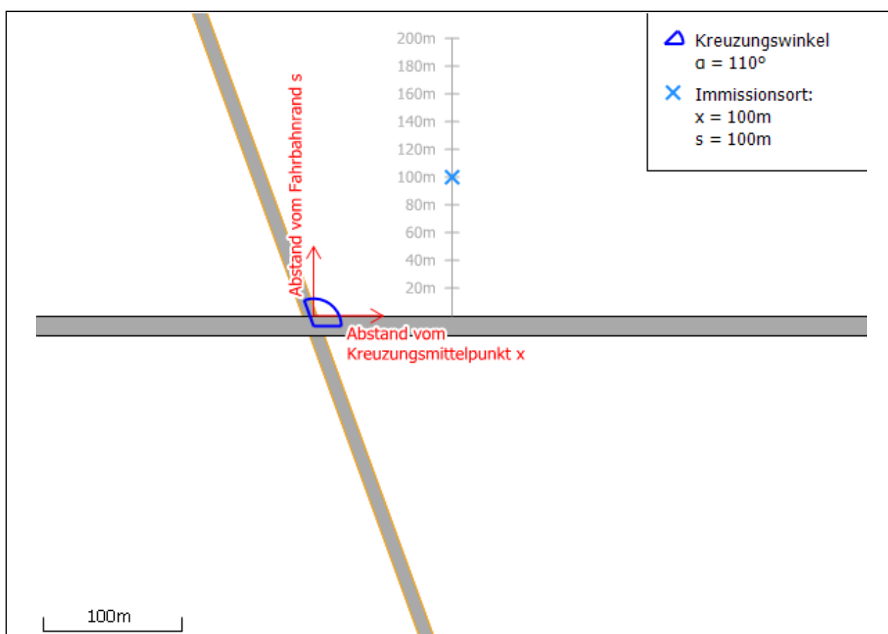
Abbildung 8: Lageplan für eine Kreuzung.
