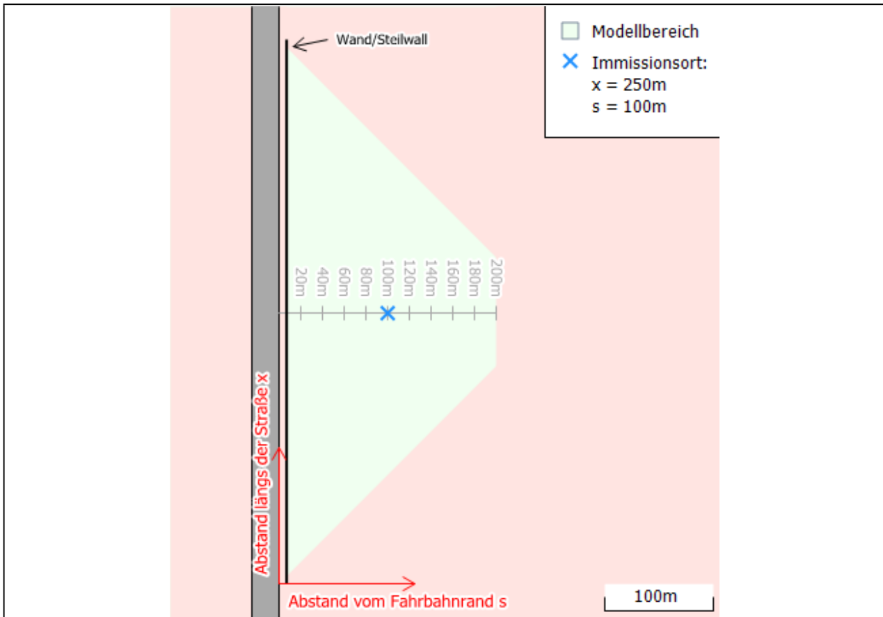
Abbildung 5: Lageplan für eine Lärmschutzmaßnahme
