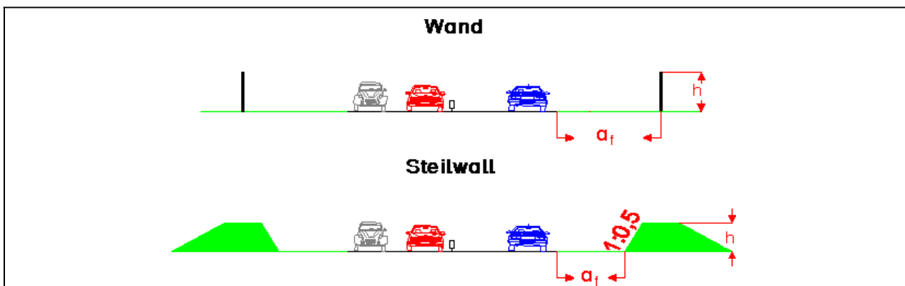
Abbildung 6: Querschnitt für Lärmschutzwand bzw. Steilwand. Lärmschutzwände/Steilwände auf beiden Straßenseiten, die immissionsseitig gleich behandelt werden.
