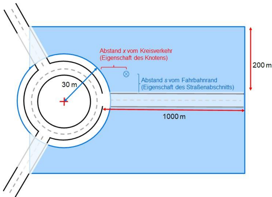
Abbildung 3: Kreisverkehrsmodul. Schematische Darstellung des Anwendungsbereiches des RLuS-Kreisverkehrsmoduls (blau ausgefüllt dargestellt) am Beispiel eines dreiarmligen Kreisverkehrs (nicht maßstabsgetreu).
