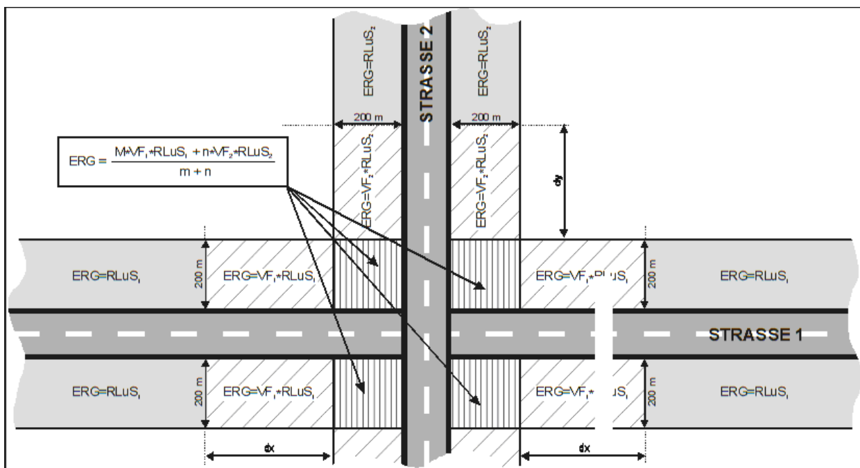
Abbildung 2: Kreuzungsmodul. Schematische Darstellung des Anwendungsbereiches des RLuS-Kreuzungsmoduls. Bei rechtwinklig schneidenden Straßen beträgt dx = dy = 800m .
